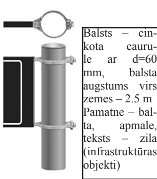
3.pielikums: Zīmes stiprinājums pie balsta (infrastruktūras objekti un māju nosaukumi)
