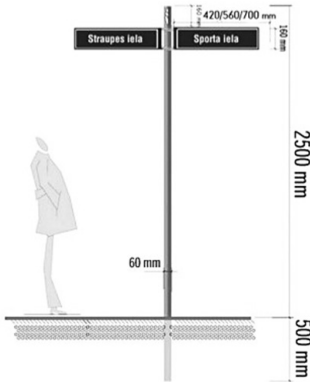
3.pielikums: Zīmes stiprinājums pie balsta (infrastruktūras objekti un māju nosaukumi)
